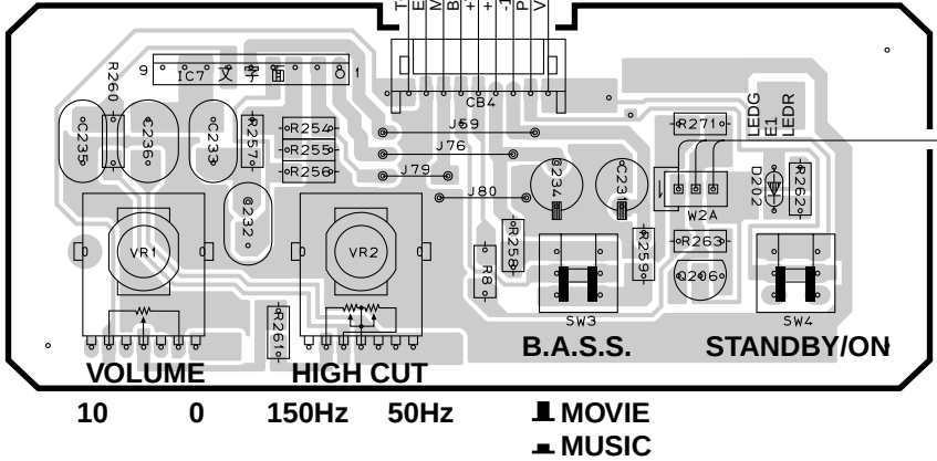
MAIN (4) P.C.B.
