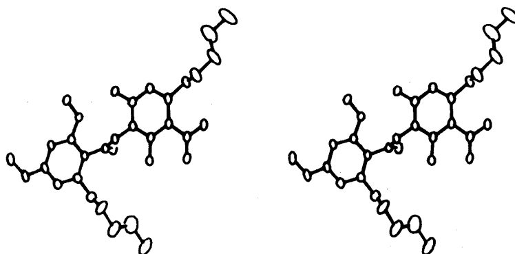
Fig. 2. ORTEP Drawing
