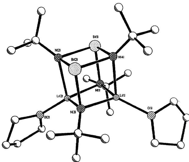
Fig. 14. Crystal structure of [\text{Bi}_2(\text{NBu}^t)_4]\text{Li}_2 \cdot 2\text{THF} ( 14 ).
