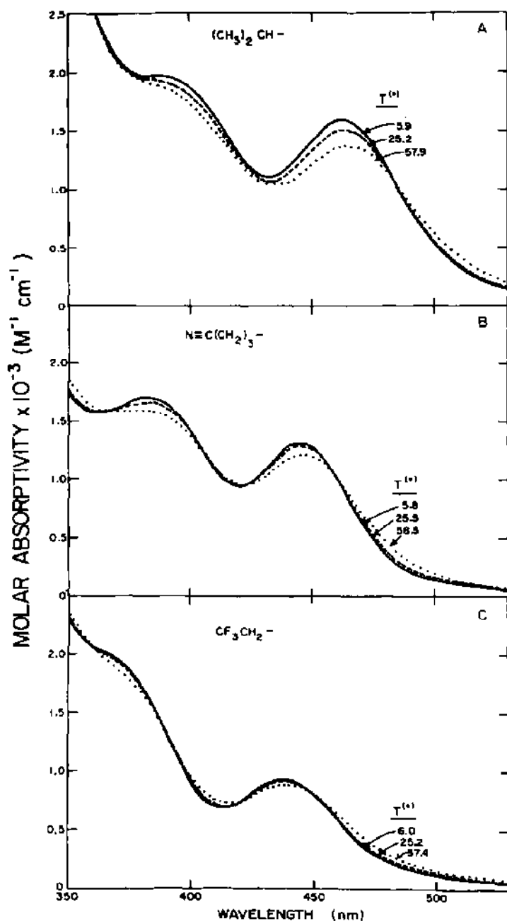
Fig. 11. Temperature dependence of the visible spectra of \text{H}_2\text{OCc}(\text{DH})_2\text{R} , pH = 6.5: (A) i\text{-C}_3\text{H}_7 , 5.9^\circ (—), 25.2^\circ (-----), 57.9^\circ (.....); (B) \text{CH}_2\text{CH}_2\text{CH}_2\text{CN} , 5.8^\circ (—), 25.5^\circ (-----), 58.5^\circ (.....); (C) \text{CH}_2\text{CF}_3 , 6.0^\circ (—), 25.2^\circ (-----), 57.4^\circ (.....). From ref. 145.
