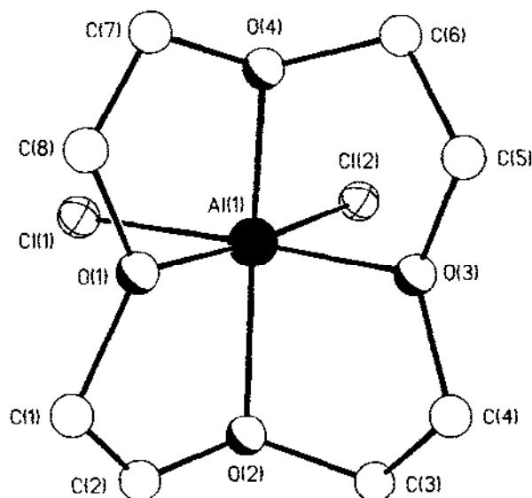
Fig. 2. View of the [12\text{-crown-4}\cdot\text{AlCl}_2]^+ cation. Selected bond distances ( \text{\AA} ) and angles (deg): \text{Al}(1)\text{--P}(1) , 1.97(1); \text{Al}(1)\text{--O}(2) , 1.97(1); \text{Al}(1)\text{--O}(3) , 1.99(1); \text{Al}(1)\text{--O}(4) , 1.92(1); \text{Al}(1)\text{--Cl}(1) , 2.202(5); \text{Al}(1)\text{--Cl}(2) , 2.200(8); \text{Cl}(2)\text{--Al}(1)\text{--Cl}(1) , 92.2(3); \text{Cl}(1)\text{--Al}(1)\text{--O}(1) , 88.0(3); \text{Cl}(2)\text{--Al}(1)\text{--O}(1) , 176.0(4); \text{Cl}(1)\text{--Al}(1)\text{--O}(2) , 97.9(4); \text{Cl}(2)\text{--Al}(1)\text{--O}(2) , 107.4(5); \text{Cl}(1)\text{--Al}(1)\text{--O}(3) , 172.3(4); \text{Cl}(2)\text{--Al}(1)\text{--O}(3) , 95.5(4); \text{Cl}(1)\text{--Al}(1)\text{--O}(4) , 99.5(4); \text{Cl}(2)\text{--Al}(1)\text{--O}(4) , 99.2(4); \text{O}(1)\text{--Al}(1)\text{--O}(2) , 76.5(5); \text{O}(1)\text{--Al}(1)\text{--O}(3) , 84.3(4); \text{O}(1)\text{--Al}(1)\text{--O}(4) , 76.8(4); \text{O}(2)\text{--Al}(1)\text{--O}(3) , 79.6(5); \text{O}(2)\text{--Al}(1)\text{--O}(4) , 147.5(5); \text{O}(3)\text{--Al}(1)\text{--O}(4) , 79.5(5).
