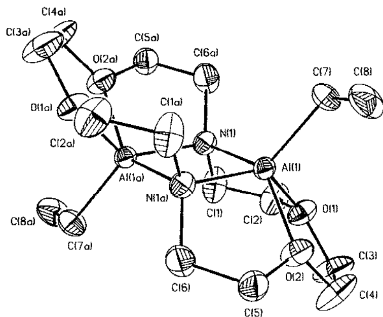
Fig. 6. View of the [\text{diaza-18-crown-6} \cdot (\text{AlEt})_2]^{2+} cation. Selected bond distances (Å) and angles (deg.): Al(1)–C(7): 1.944(5); Al(1)–O(1): 1.950(5); Al(1)–O(2): 1.959(5); Al(1)–N(1): 1.972(3); Al(1)–N(1a): 1.963(4); Al(1)–Al(1a): 2.902(3); C(7)–Al(1)–N(1): 114.5(2); C(7)–Al(1)–N(1a): 117.1(2); C(7)–Al(1)–O(1): 108.9(2); C(7)–Al(1)–O(2): 106.3(2); O(1)–Al(1)–N(1): 82.9(2); O(1)–Al(1)–O(2): 76.9(2); N(1)–Al(1)–N(1a): 85.0(2); O(2)–Al(1)–N(1a): 83.3(2); Al(1)–C(7)–C(8): 117.2(5).
