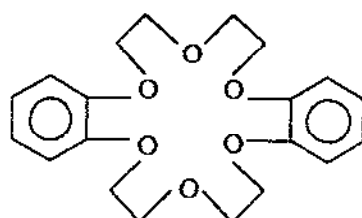
dibenzo-18-crown-6
