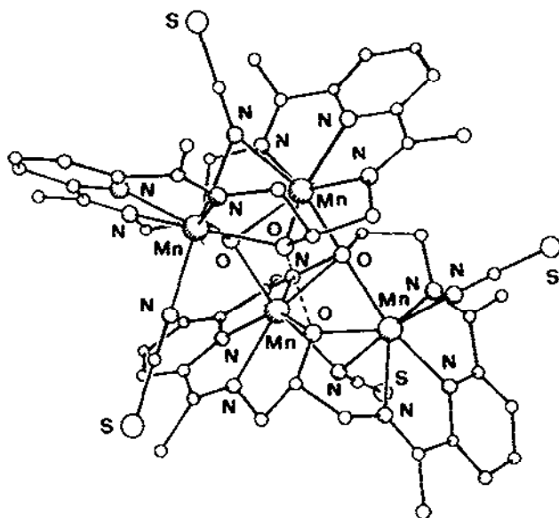
Fig. 105. Structure of [\text{Mn}_4(45-2H)(45-H)(\text{NCS})_4]^+ .
