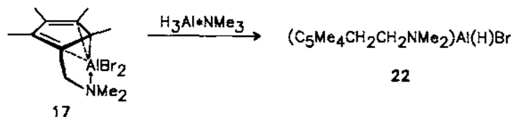
Scheme 14.
