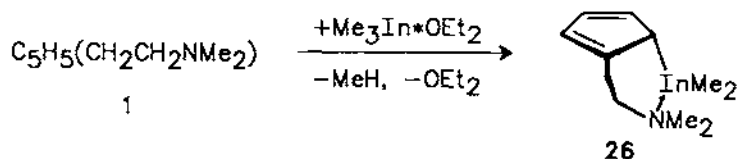
Scheme 17.
