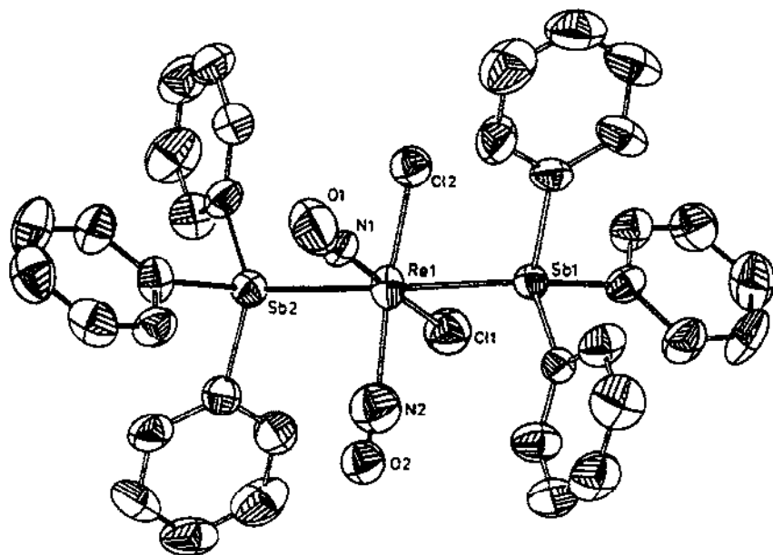
Fig. 5. Molecular structure of \text{ReCl}_2(\text{NO})_2(\text{Ph}_3\text{Sb})_2 . (From ref. 296 by permission of Zeitschrift für Anorganische und Allgemeine Chemie .)
