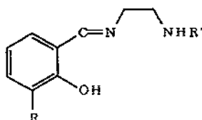
HRSalR'en
