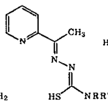
HAT
