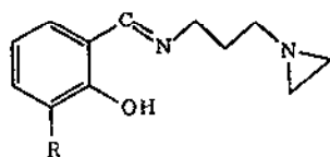
HSalAPA
