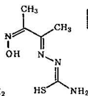
HDMT
