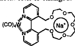
W(CO) 4 -(1)
