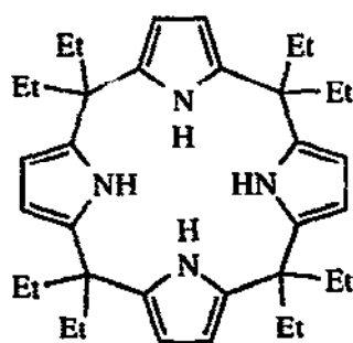
H 4 Et 8 P (21)
