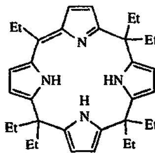
H 3 Et 7 P (22)
