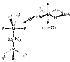
(\eta^2\text{-BH}_4)_2\text{Zr}(\mu_2\text{-H})_2\text{Zr}(\text{PMe}_3)_2(\eta^2\text{-BH}_4)_2 [64]
