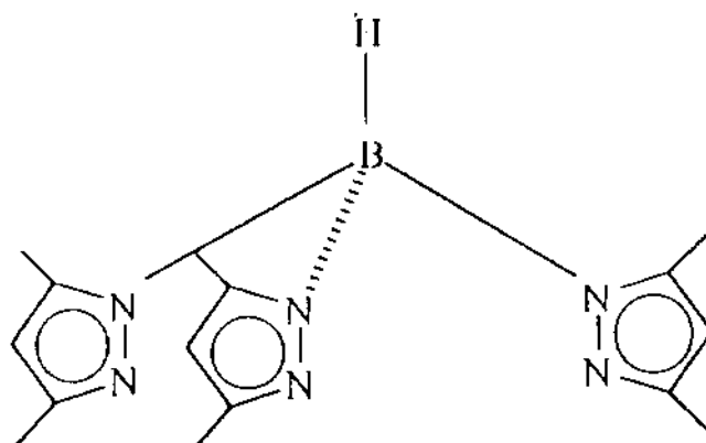
Fig. 11. A tris-pyrazolylborate ligand.
