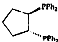
12 = ( R )-DPPCP
