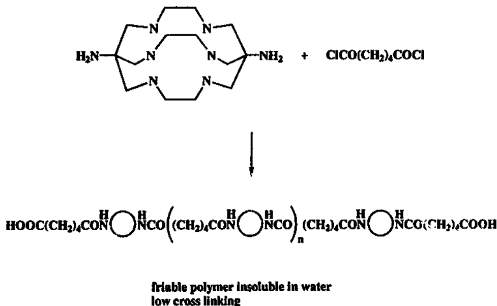
Fig. 10. Cage polymer.
