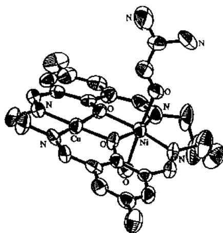
[CuNi(L^4)(H_2O)(dmf)]^{2+}
