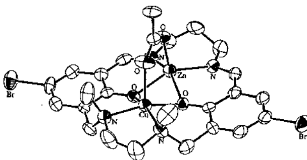
[CuNi(L 8 )(AcO)] +
