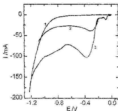
Fig. 1. Voltammetric curves in the \text{KF}\cdot\text{K}_2\text{MoO}_4\text{--B}_2\text{O}_3 system: (1) Pure \text{K}_2\text{MoO}_4 ; (2) \text{K}_2\text{MoO}_4\text{--}2 \text{ mol\% B}_2\text{O}_3 ; (3) \text{K}_2\text{MoO}_4\text{--}5 \text{ mol\% B}_2\text{O}_3 .
