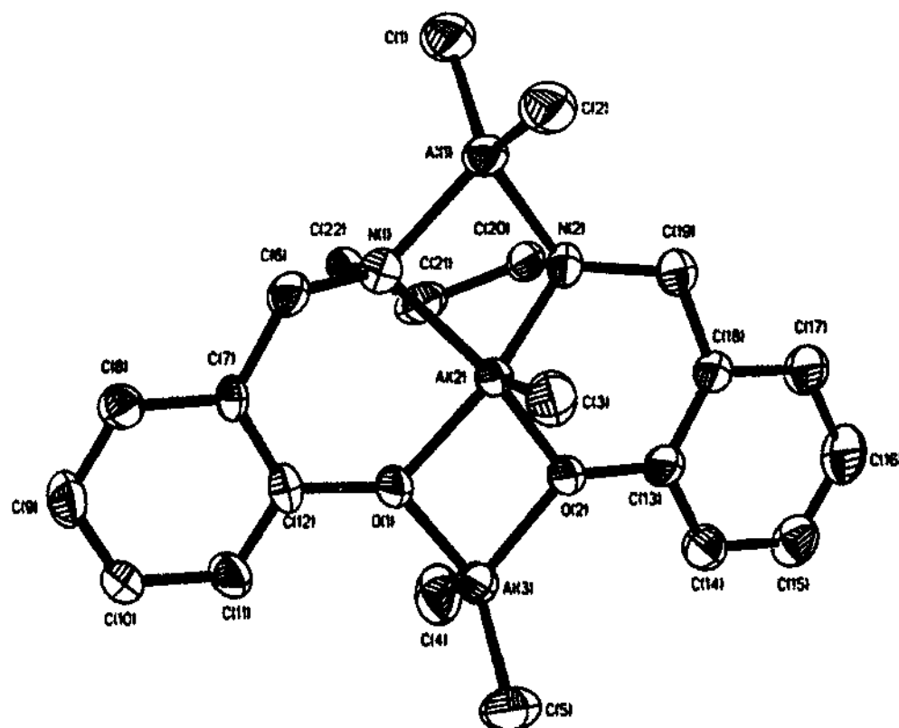
Fig. 18. Molecular structure of SalpanAlMe(AlMe 2 ) 2 ( 32 ).
