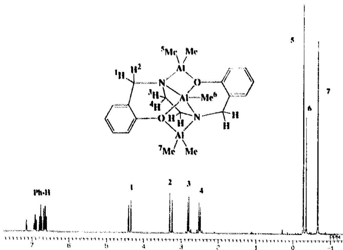
Fig. 12. 1 H NMR spectrum of SaleanAlMe(AlMe 2 ) 2 ( 29 )
