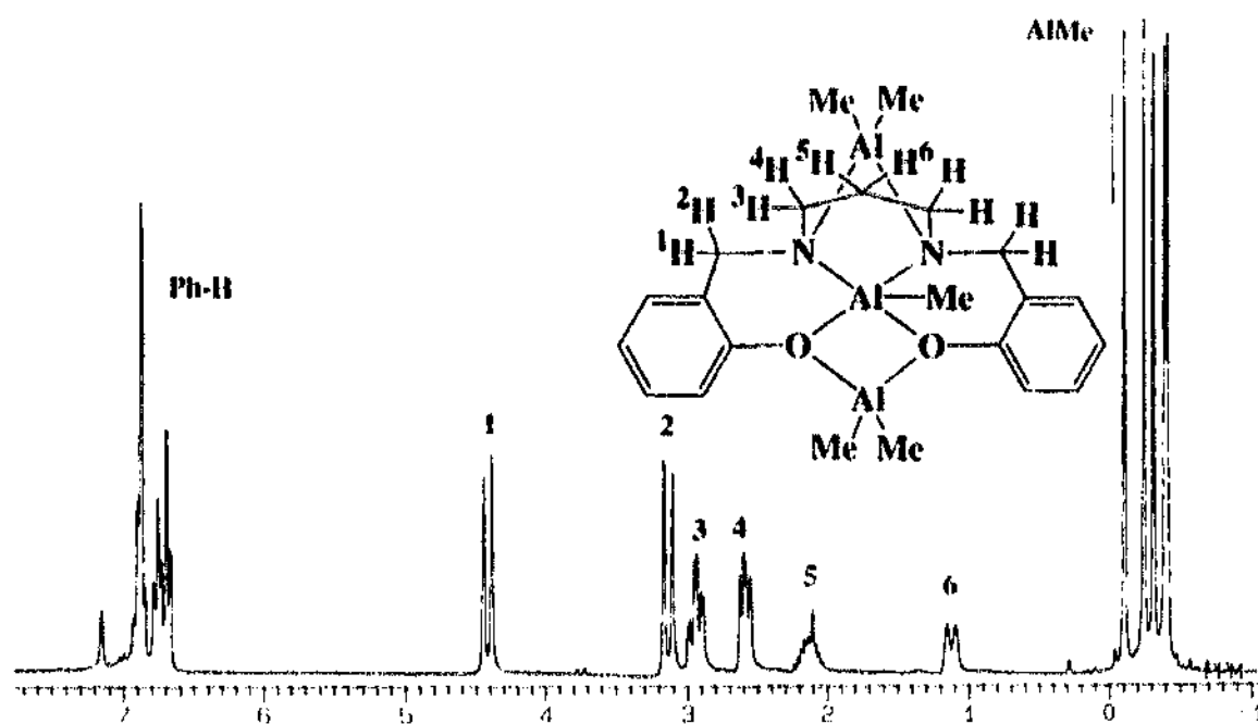
Fig. 13. 1 H NMR spectrum of SalpanAlMe(AlMe 2 ) 2 (32).
