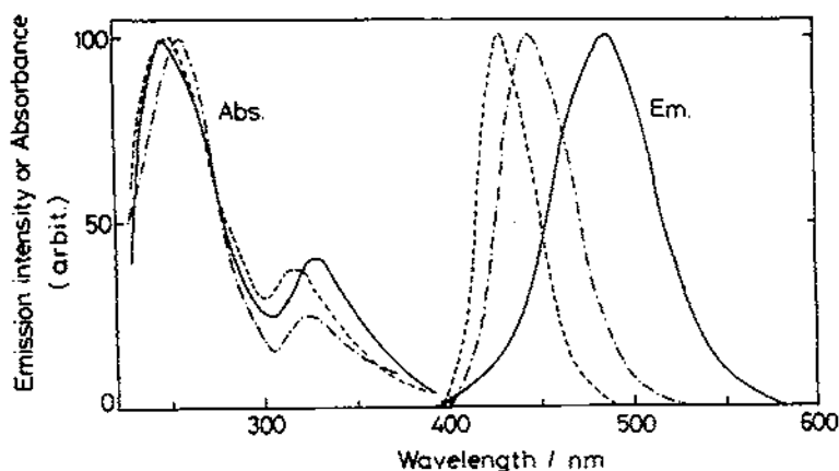
Fig. 3. The emission and absorption spectra of \text{Eu}^{2+} -15C5 (---), \text{Eu}^{2+} -18C6 complex (- · -), and \text{EuCl}_2 (—) in methanol.
