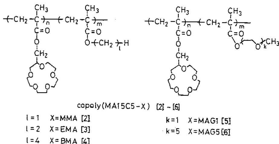
Scheme 3. Schematic structure of the 15C5 copolymer: (a) l=1 , X=\text{MMA} ; (b) l=2 , X=\text{EMA} ; (c) l=4 , X=\text{BMA} ; (d) k=1 , X=\text{MAG1} ; (e) k=5 , X=\text{MAG5} .
