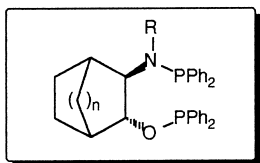
n = 0, R = H AC-PONP n = 0, R = Me MAC-PONP n = 1, R = Me
