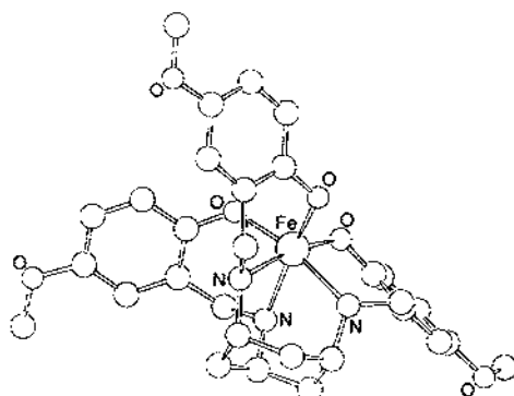
[Fe(208)]
