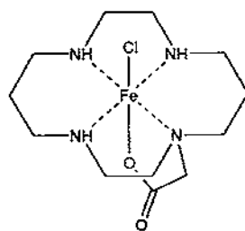
( 243 )
