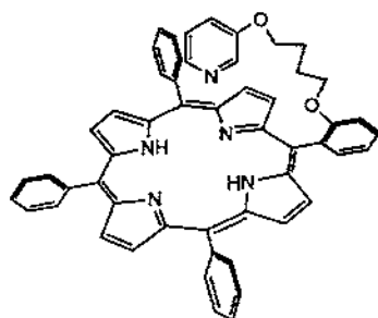
\text{H}_2(93)
