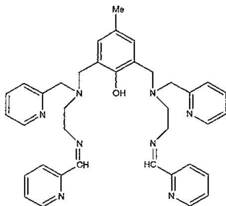
H-(272)
