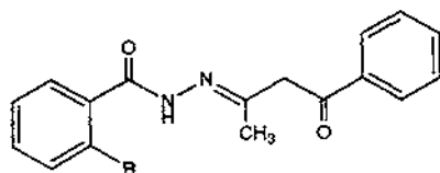
( 244 ) R=H ( 245 ) R=OH
