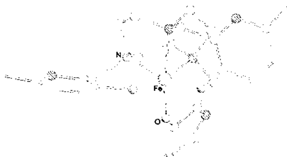
[Fe(265)]
