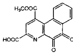
H-(237)
