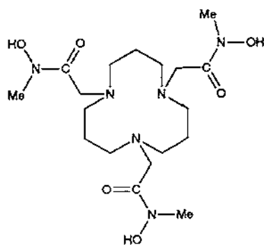
H_3 –(266)
