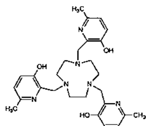
H_3 –(265)
