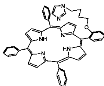
\text{H}_2(94)
