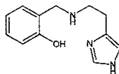
H(216)
