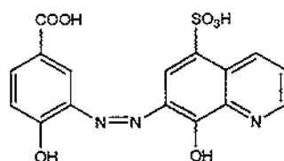
H_4 -( 241 )
