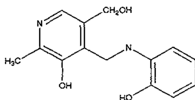
H-(239)
