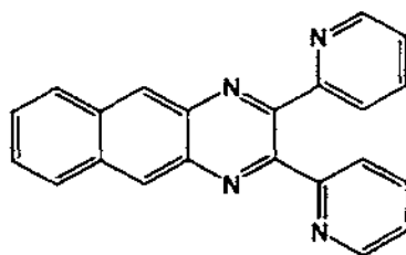
(25)
