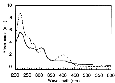
Fig. 5. UV-Vis spectra of Salpr-MTS (---) and Mn(II)Salpr-MTS (—).
