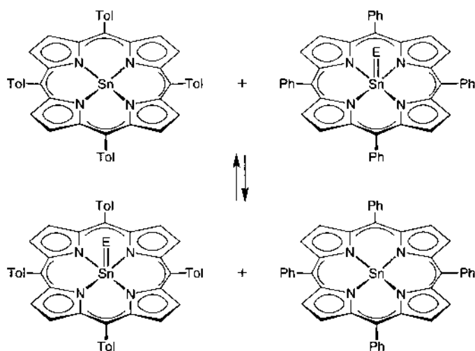
Scheme 30.
