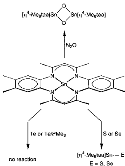
Scheme 18.
