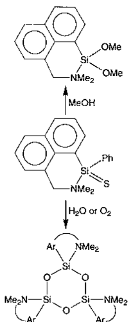
Scheme 27.
