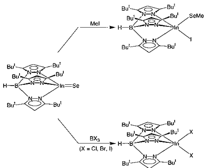
Scheme 24.
