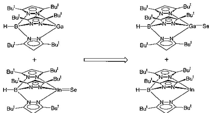
Scheme 22.
