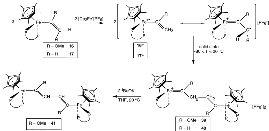
Scheme 18.
