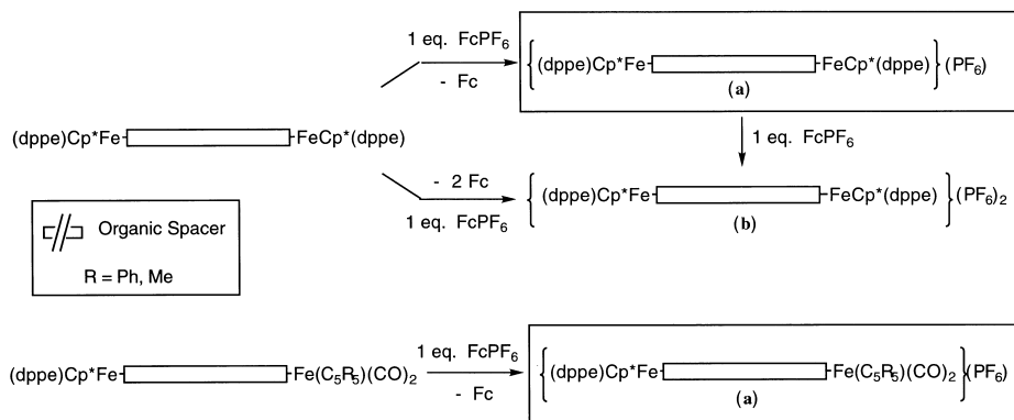
Scheme 20.
