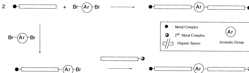
Scheme 17.
