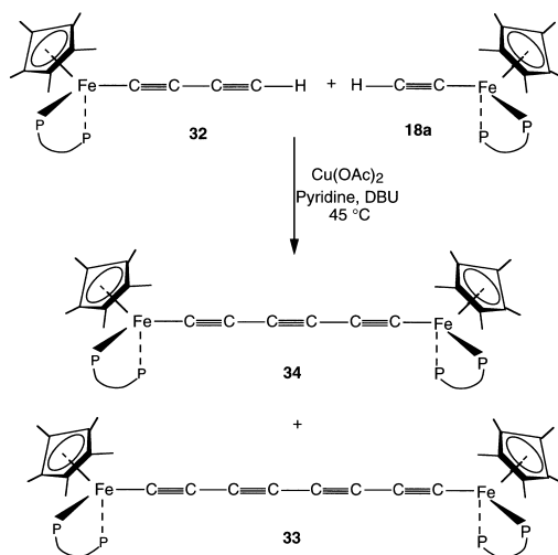
Scheme 14.
