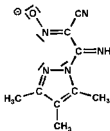
9: \{\text{tmpz.ONC(CN)}_2\}^-
