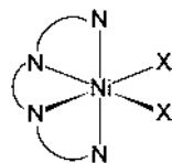
cis - α
