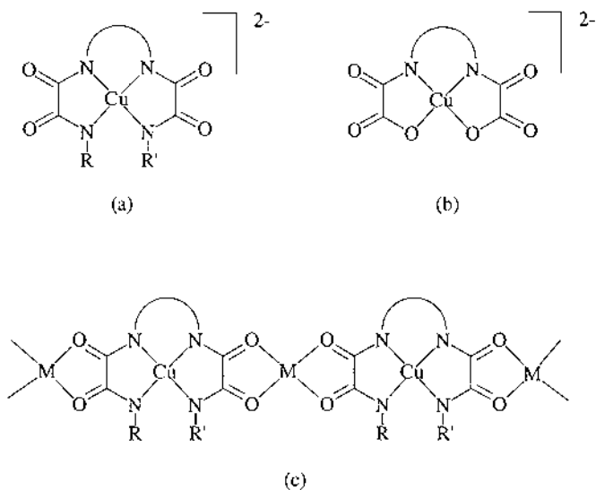
Scheme 14.
