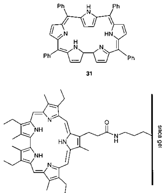
Fig. 5. Sapphyrin modified silica gel.
