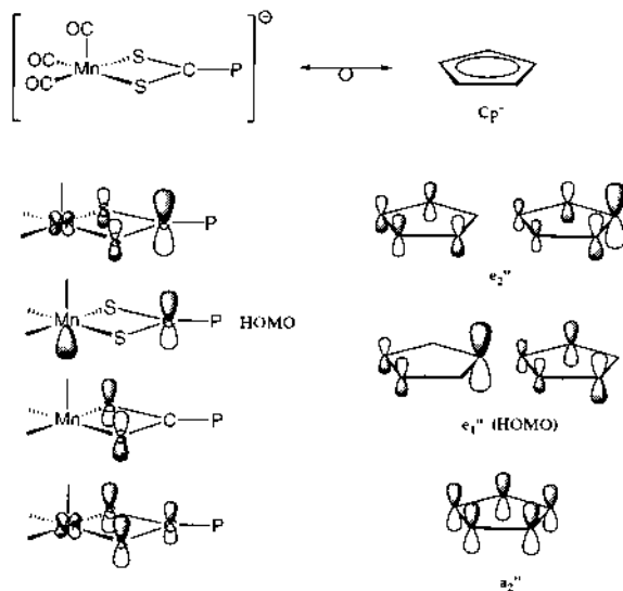
Scheme 19.
