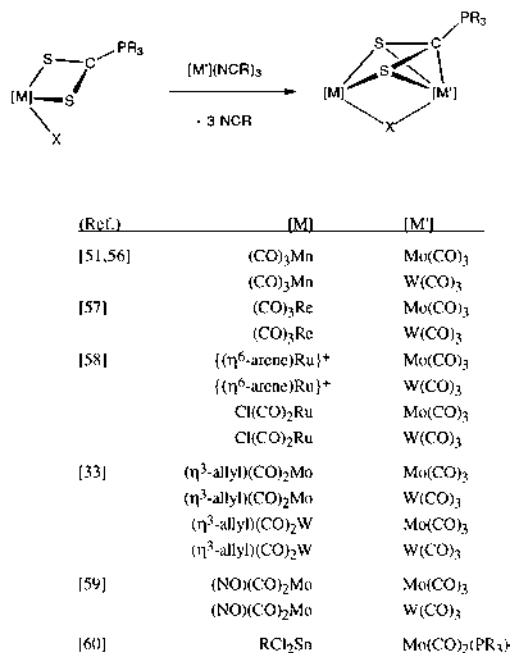
Scheme 17.
