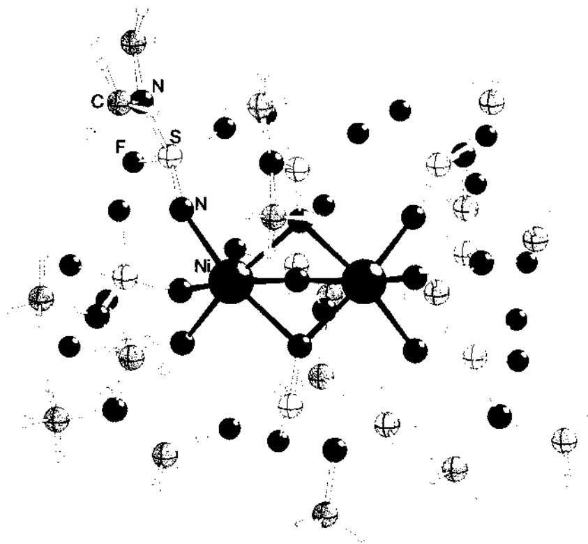
Fig. 28. Crystal structure of [\text{Ni}_2(\text{NSF}_2\text{NMe}_2)_9](\text{AsF}_6)_4 [128].
