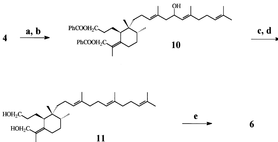
Scheme 3. Synthesis of 10-desoxyiridal 6 . Reagents: (a) NaBH 4 , (b) PhCOCl, pyridine, (c) Ph 3 PBr 2 , (d) LiAlH 4 and (e) MnO 2 .
