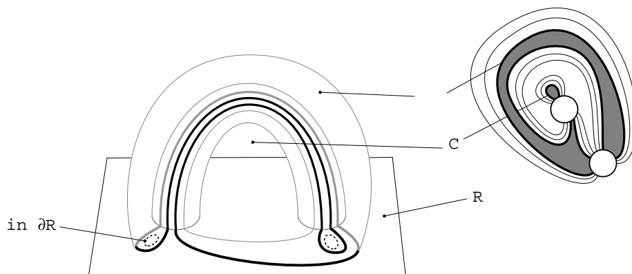
FIGURE 23. R \cup S \cup C \cup C_2
