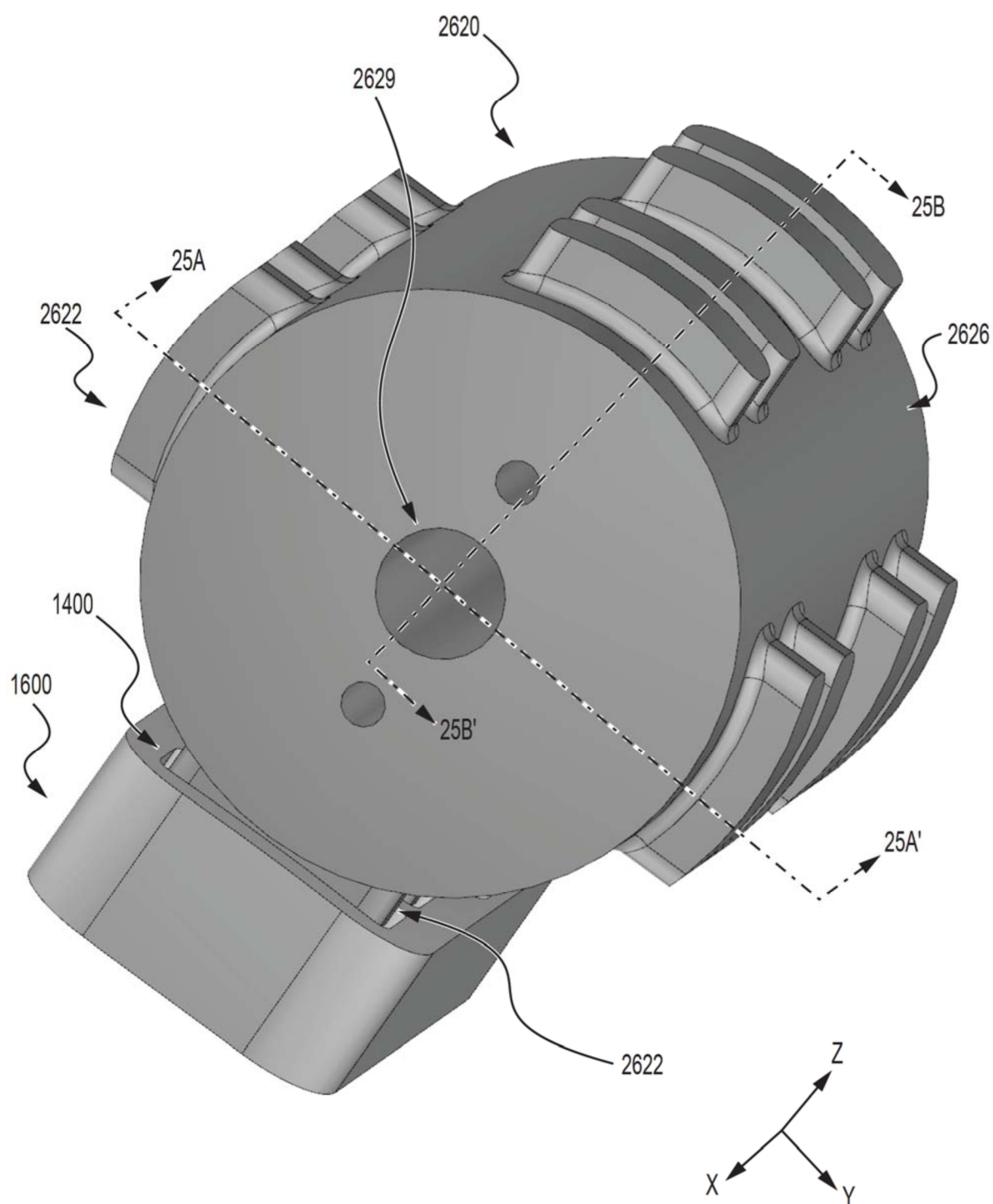
FIG. 22A
