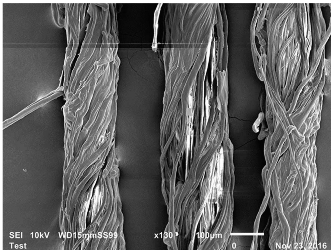
FIG. 9J
