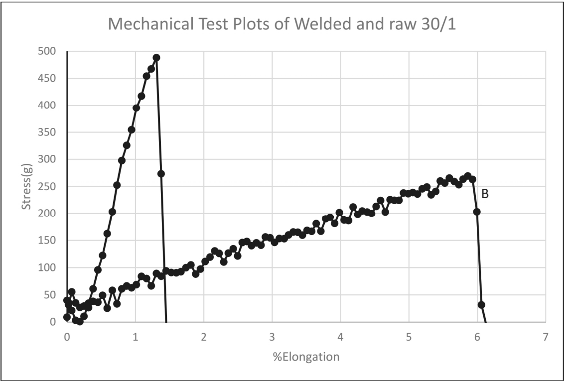
FIG. 10G
